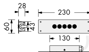
Externes Schaltelement mit 5 Wippschalter
