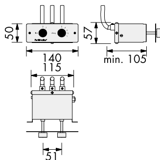
Externes Schaltelement mit 2 Drehschalter
